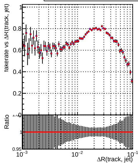
—•— DQM_CKF_XiMinusNOPU_base —•— DQM_CKF_XiMinusNOPU_retrainOldFiles125_v2_prelimWPM_epoch2
