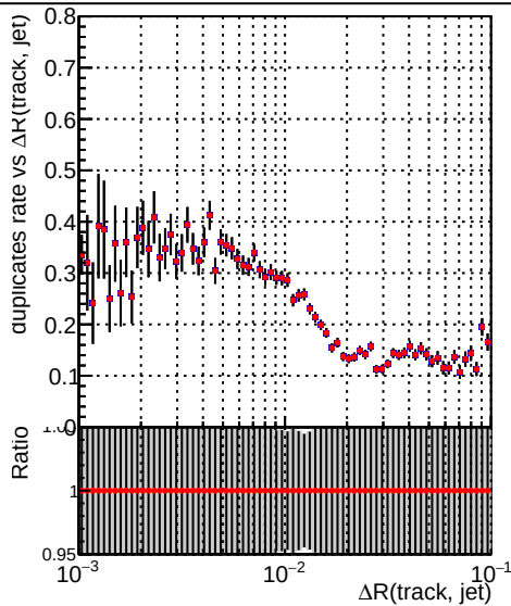
—•— DQM_CKF_XiMinusNOPU_base —•— DQM_CKF_XiMinusNOPU_retrainOldFiles125_v2_prelimWPM_epoch2
