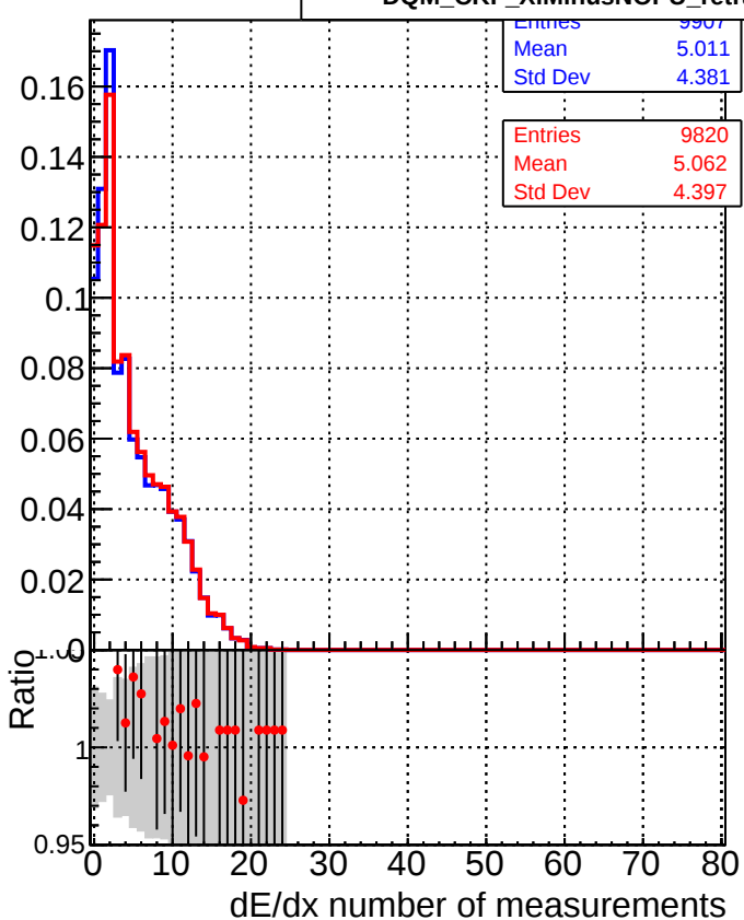
—■— DQM_CKF_XiMinusNOPU_base —●— DQM_CKF_XiMinusNOPU_retrainOldFiles125_v2_prelimWPM_epoch2
