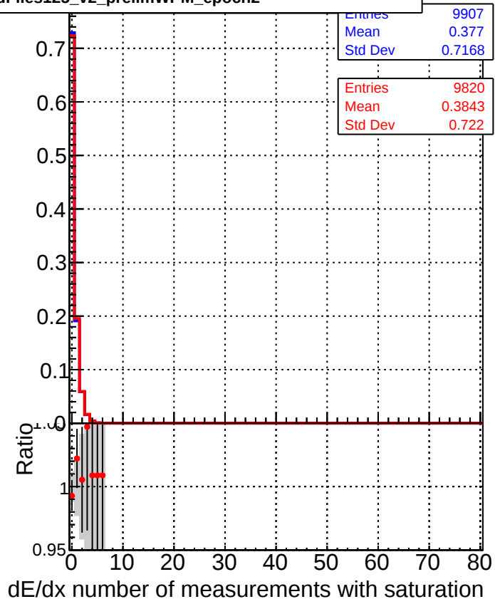
—■— DQM_CKF_XiMinusNOPU_base —●— DQM_CKF_XiMinusNOPU_retrainOldFiles125_v2_prelimWPM_epoch2
