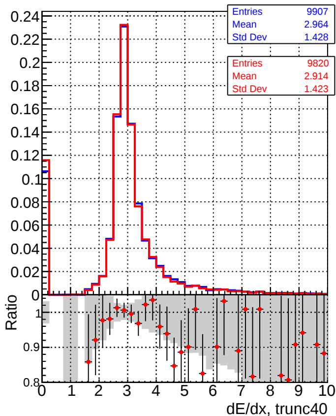
—■— DQM_CKF_XiMinusNOPU_base —●— DQM_CKF_XiMinusNOPU_retrainOldFiles125_v2_prelimWPM_epoch2
