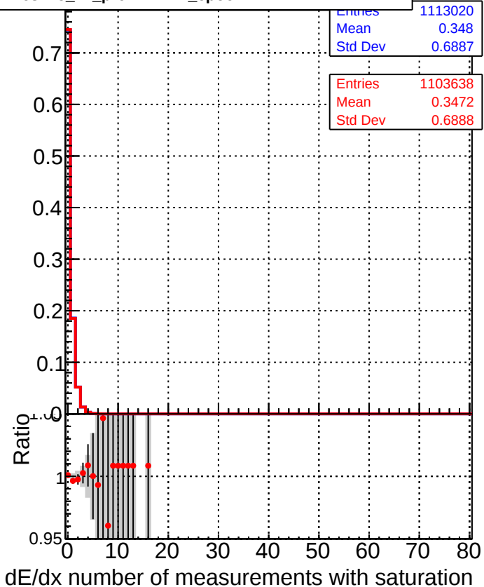
—■— DQM_CKF_XiMinusNOPU_base —●— DQM_CKF_XiMinusNOPU_retrainOldFiles125_v2_prelimWPM_epoch2
