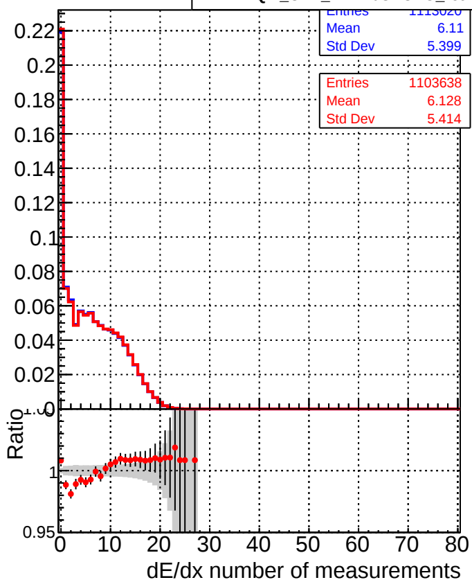
—■— DQM_CKF_XiMinusNOPU_base —●— DQM_CKF_XiMinusNOPU_retrainOldFiles125_v2_prelimWPM_epoch2
