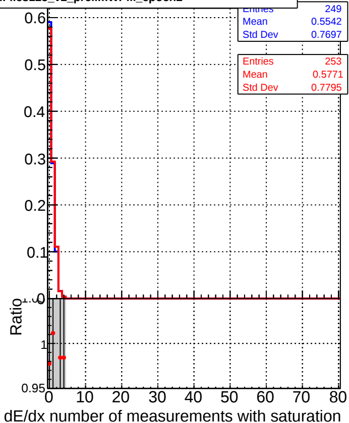
■ DQM_CKF_XiMinusNOPU_base ● DQM_CKF_XiMinusNOPU_retrainOldFiles125_v2_prelimWPM_epoch2
