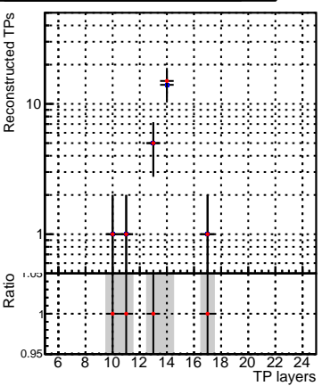
■ DQM_CKF_XiMinusNOPU_base ■ DQM_CKF_XiMinusNOPU_retrainOldFiles125_v2_prelimWPM_epoch2
