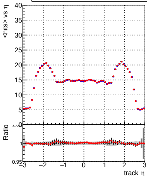
mean hits — DQM_CKF_XiMinusNOPU_base — DQM_CKF_XiMinusNOPU_retrainOldFiles125_v2_prelimWPM_epoch2
