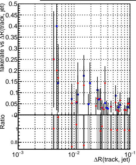
—●— DQM_CKF_XiMinusNOPU_base —●— DQM_CKF_XiMinusNOPU_retrainOldFiles125_v2_prelimWPM_epoch2
