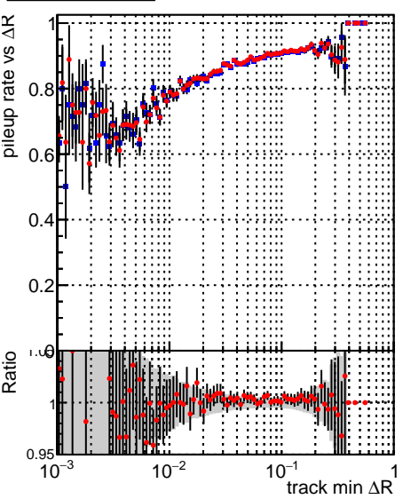
—●— DQM_CKF_XiMinusNOPU_base —●— DQM_CKF_XiMinusNOPU_retrainOldFiles125_v2_prelimWPM_epoch2
