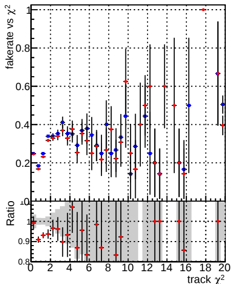
Fake rate vs. —◆— DQM CKF XMinusNOPU_base —●— DQM CKF XMinusNOPU_retrainOldFiles125_v2_prelimWPM_epoch2
