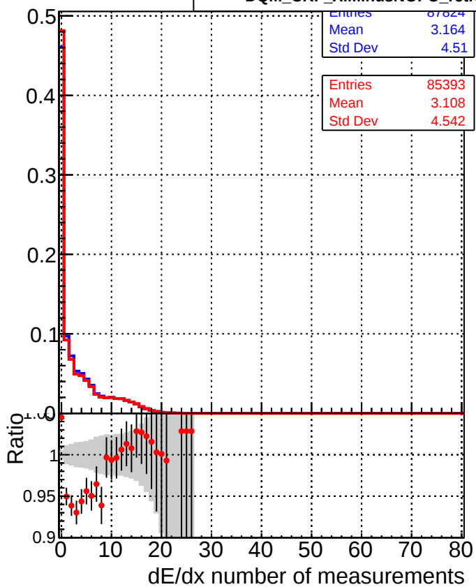
■ DQM_CKF_XiMinusNOPU_base ● DQM_CKF_XiMinusNOPU_retrainOldFiles125_v2_prelimWPM_epoch2
