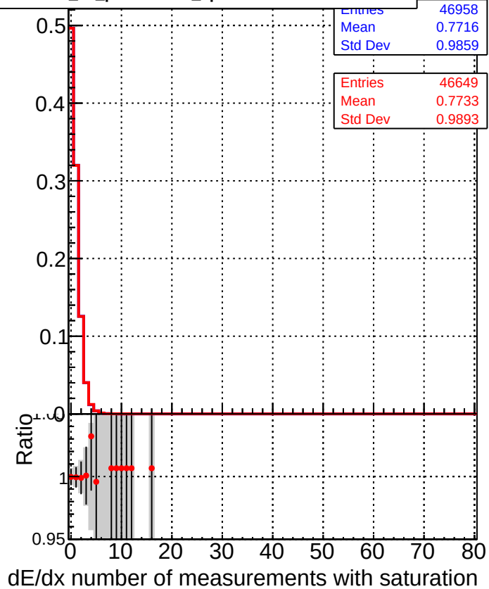
DQM_CKF_XiMinusNOPU_base DQM_CKF_XiMinusNOPU_retrainOldFiles125_v2_prelimWPM_epoch2
