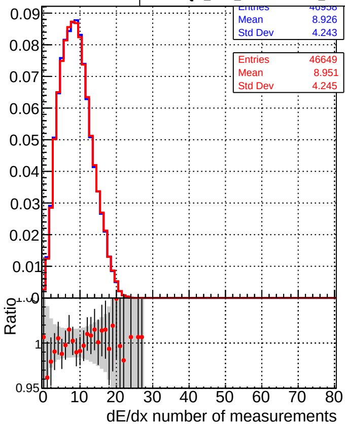
DQM_CKF_XiMinusNOPU_base DQM_CKF_XiMinusNOPU_retrainOldFiles125_v2_prelimWPM_epoch2
