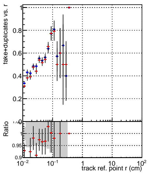
■ DQM_CKF_XiMinusNOPU_base ● DQM_CKF_XiMinusNOPU_retrainOldFiles125_v2_prelimWPM_epoch2
