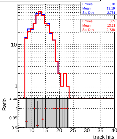
DQM_CKF_XiMinusNOPU_retrainOldFiles125_v2_prelimWPM_epoch2
