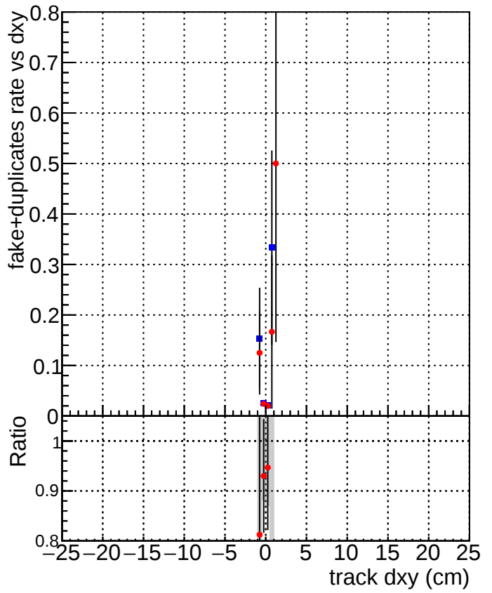
DQM_CKF_XiMinusNOPU_base DQM_CKF_XiMinusNOPU_retrainOldFiles125_v2_prelimWPM_epoch2
