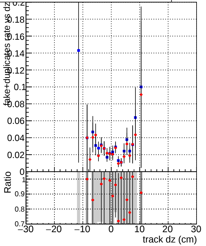
DQM_CKF_XiMinusNOPU_base DQM_CKF_XiMinusNOPU_retrainOldFiles125_v2_prelimWPM_epoch2
