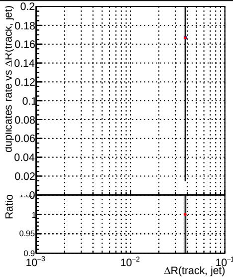
—●— DQM_CKF_XiMinusNOPU_base —●— DQM_CKF_XiMinusNOPU_retrainOldFiles125_v2_prelimWPM_epoch2
