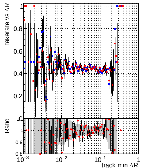
—●— DQM_CKF_XiMinusNOPU_base —●— DQM_CKF_XiMinusNOPU_retrainOldFiles125_v2_prelimWPM_epoch2
