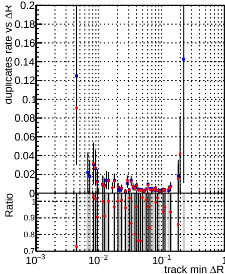
—●— DQM_CKF_XiMinusNOPU_base —●— DQM_CKF_XiMinusNOPU_retrainOldFiles125_v2_prelimWPM_epoch2
