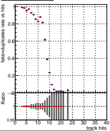
■ DQM_CKF_XiMinusNOPU_base ● DQM_CKF_XiMinusNOPU_retrainOldFiles125_v2_prelimWPM_epoch2
