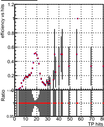
■ DQM_CKF_XiMinusNOPU_base ● DQM_CKF_XiMinusNOPU_retrainOldFiles125_v2_prelimWPM_epoch2
