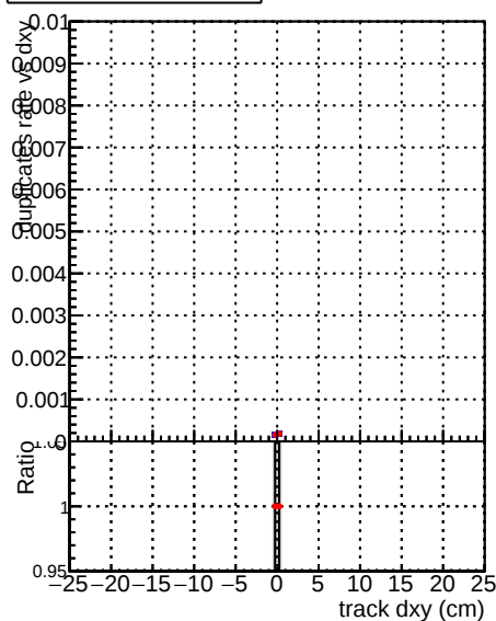
—●— DQM_CKF_XiMinusNOPU_base —●— DQM_CKF_XiMinusNOPU_retrainOldFiles125_v2_prelimWPM_epoch2
