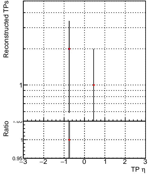
—●— DQM_CKF_XiMinusNOPU_base —●— DQM_CKF_XiMinusNOPU_retrainOldFiles125_v2_prelimWPM_epoch2
