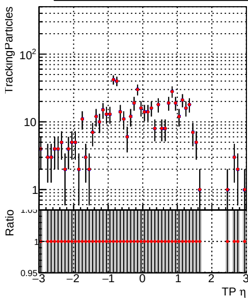
—•— DQM_CKF_XiMinusNOPU_base —•— DQM_CKF_XiMinusNOPU_retrainOldFiles125_v2_prelimWPM_epoch2
