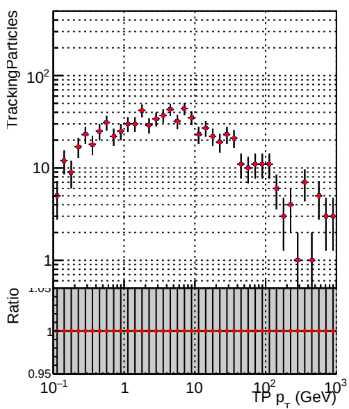
—•— DQM_CKF_XiMinusNOPU_base —•— DQM_CKF_XiMinusNOPU_retrainOldFiles125_v2_prelimWPM_epoch2
