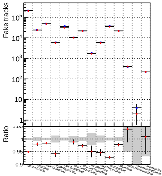
DQM_CKF_XiMinusNOPU_retrainOldFiles125_v2_prelimWPM_epoch2
