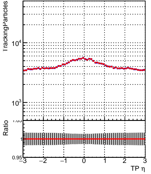
—■ DQM_CKF_XiMinusNOPU_base —■ DQM_CKF_XiMinusNOPU_retrainOldFiles125_v2_prelimWPM_epoch2
