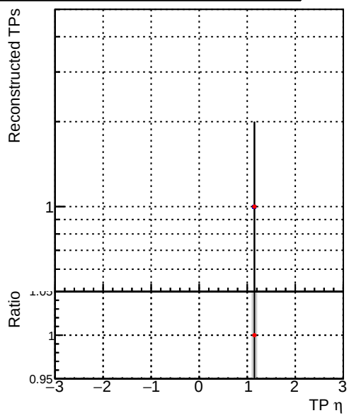
—●— DQM_CKF_XiMinusNOPU_base —●— DQM_CKF_XiMinusNOPU_retrainOldFiles125_v2_prelimWPM_epoch2
