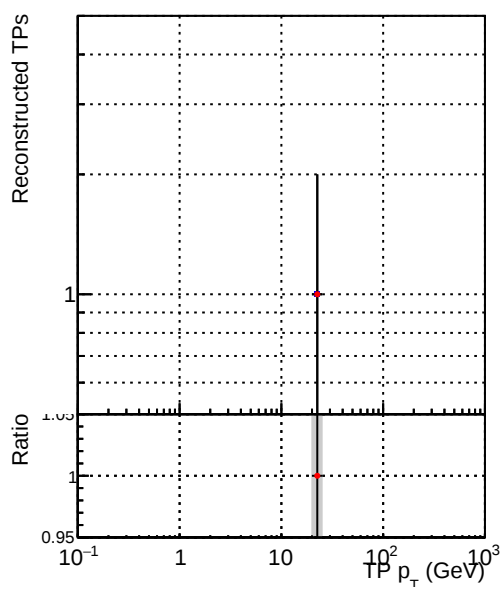
—●— DQM_CKF_XiMinusNOPU_base —●— DQM_CKF_XiMinusNOPU_retrainOldFiles125_v2_prelimWPM_epoch2
