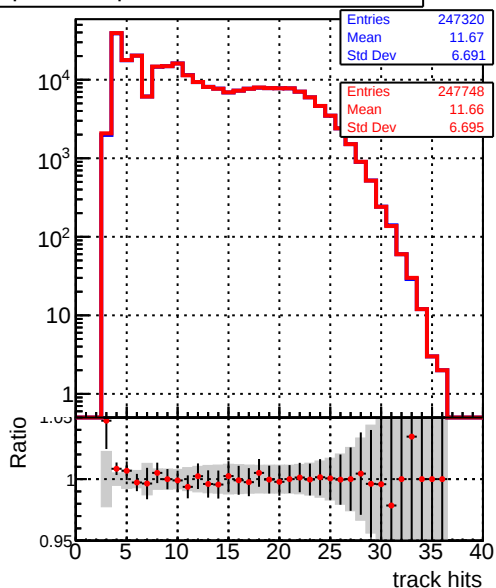
DQM_CKF_XiMinusNOPU_retrainOldFiles125_v2_prelimWPM_epoch2
