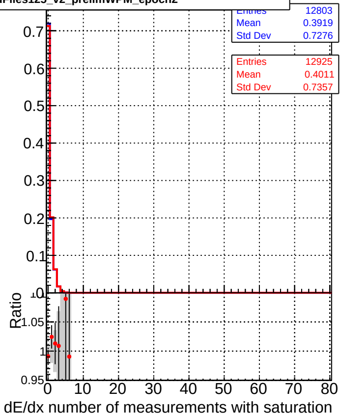
—■— DQM_CKF_XiMinusNOPU_base —●— DQM_CKF_XiMinusNOPU_retrainOldFiles125_v2_prelimWPM_epoch2
