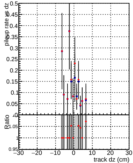
DQM CKF_XiMinusNOPU_retrainOldFiles125_v2_prelimWPM_epoch2
