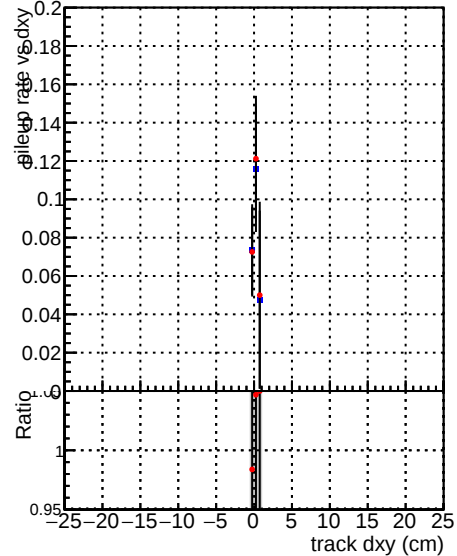
DQM CKF_XiMinusNOPU_retrainOldFiles125_v2_prelimWPM_epoch2
