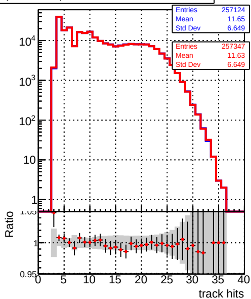
DQM_CKF_XiMinusNOPU_retrainOldFiles125_v2_prelimWPM_epoch2
