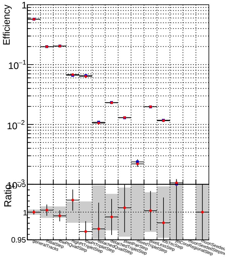
DQM_CKF_XiMinusNOPU_base DQM_CKF_XiMinusNOPU_retrainOldFiles125_v2_prelimWPM_epoch1
