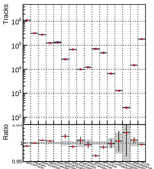
DQM_CKF_XiMinusNOPU_base
