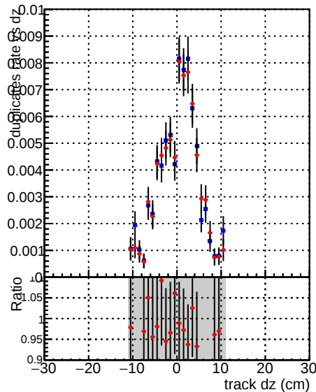
DQM CKF XiMinusNOPU_base
