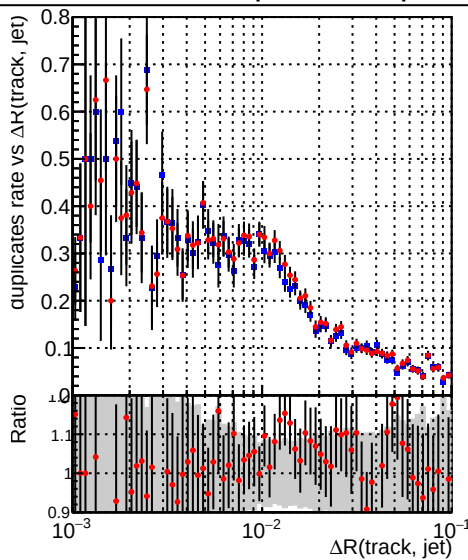
■ DQM_CKF_XiMinusNOPU_base ● DQM_CKF_XiMinusNOPU_retrainOldFiles125_v2_prelimWPM_epoch1
