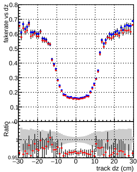
—●— DQM CKF XiMinusNOPU_base —●— DQM CKF XiMinusNOPU_retrainOldFiles125_v2_prelimWPM_epoch1
