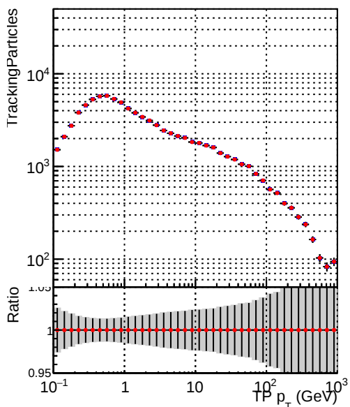
—•— DQM_CKF_XiMinusNOPU_base —•— DQM_CKF_XiMinusNOPU_retrainOldFiles125_v2_prelimWPM_epoch1
