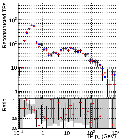
—•— DQM_CKF_XiMinusNOPU_base —•— DQM_CKF_XiMinusNOPU_retrainOldFiles125_v2_prelimWPM_epoch1
