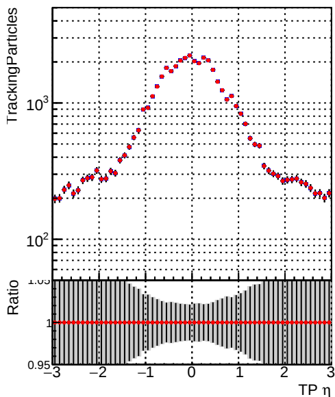
—•— DQM_CKF_XiMinusNOPU_base —•— DQM_CKF_XiMinusNOPU_retrainOldFiles125_v2_prelimWPM_epoch1
