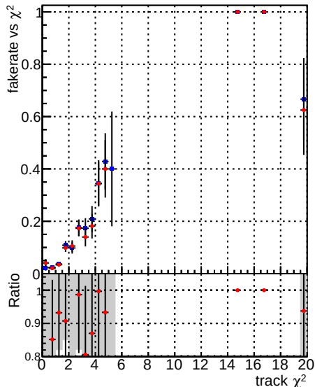
Fake rate vs. ◆ DQM CKF XiMinusNOPU_base ▲ DQM CKF XiMinusNOPU_retrainOldFiles125_v2_prelimWPM_epoch1
