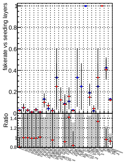
Fake rate vs. ◆ DQM CKF XiMinusNOPU_base ▲ DQM CKF XiMinusNOPU_retrainOldFiles125_v2_prelimWPM_epoch1
