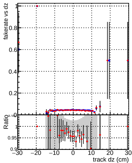
Fake rate vs d DQM CKF XiMinusNOPU_base DQM CKF XiMinusNOPU_retrainOldFiles125_v2_prelimWPM_epoch1
