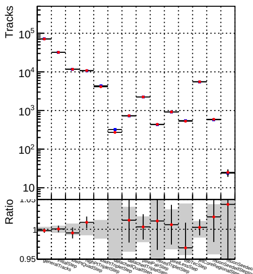
DQM_CKF_XiMinusNOPU_base
