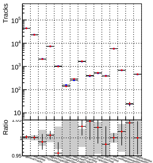
■ DQM_CKF_XiMinusNOPU_base
