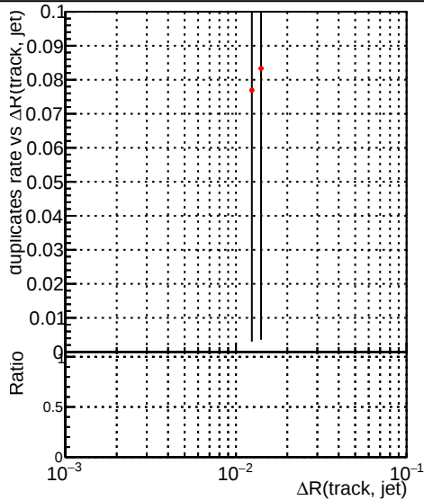
—●— DQM_CKF_XiMinusNOPU_base —●— DQM_CKF_XiMinusNOPU_retrainOldFiles125_v2_prelimWPM_epoch1
