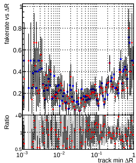
—●— DQM_CKF_XiMinusNOPU_base —●— DQM_CKF_XiMinusNOPU_retrainOldFiles125_v2_prelimWPM_epoch1
