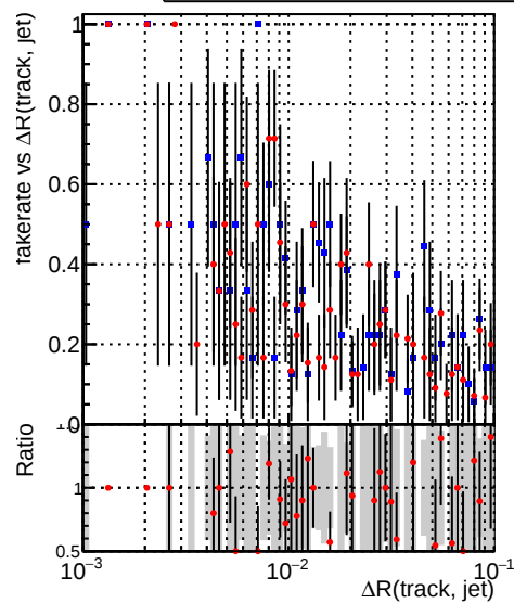
—●— DQM_CKF_XiMinusNOPU_base —●— DQM_CKF_XiMinusNOPU_retrainOldFiles125_v2_prelimWPM_epoch1
