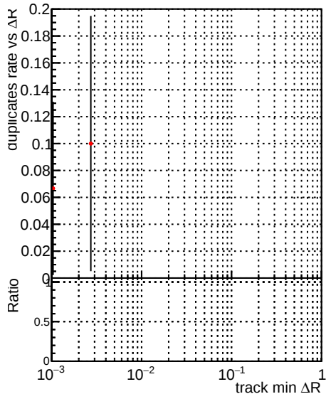
—●— DQM_CKF_XiMinusNOPU_base —●— DQM_CKF_XiMinusNOPU_retrainOldFiles125_v2_prelimWPM_epoch1
