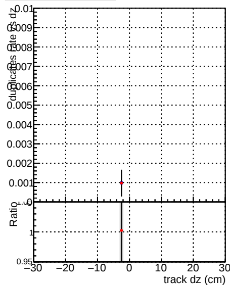
—●— DQM_CKF_XiMinusNOPU_base —●— DQM_CKF_XiMinusNOPU_retrainOldFiles125_v2_prelimWPM_epoch1
