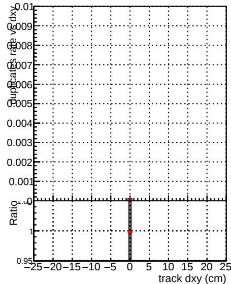
—●— DQM_CKF_XiMinusNOPU_base —●— DQM_CKF_XiMinusNOPU_retrainOldFiles125_v2_prelimWPM_epoch1
