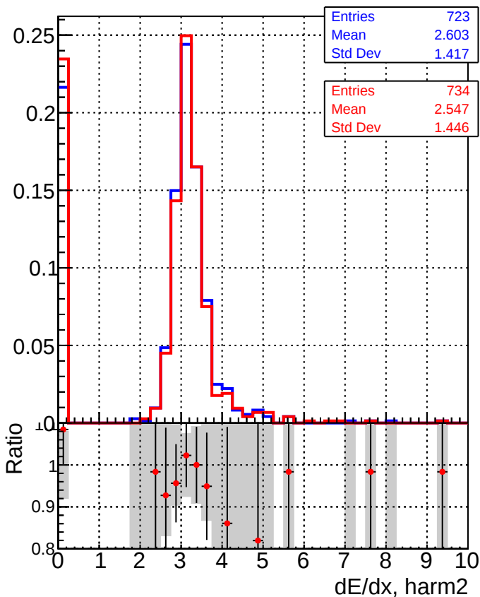
■ DQM_CKF_XiMinusNOPU_base ● DQM_CKF_XiMinusNOPU_retrainOldFiles125_v2_prelimWPM_epoch1
