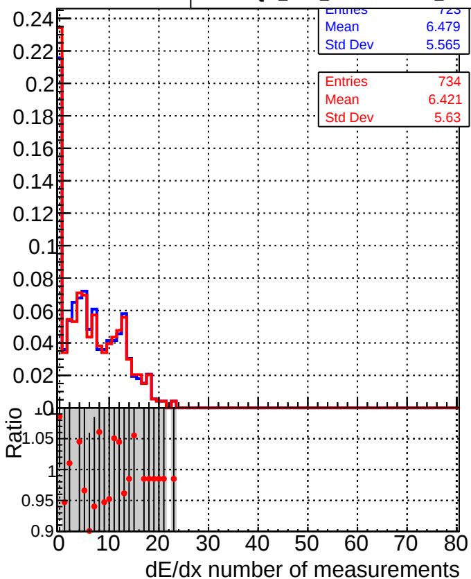
■ DQM_CKF_XiMinusNOPU_base ● DQM_CKF_XiMinusNOPU_retrainOldFiles125_v2_prelimWPM_epoch1
