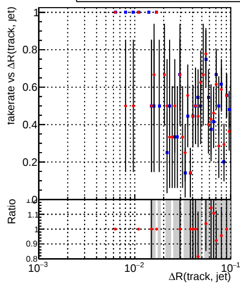
—•— DQM_CKF_XiMinusNOPU_base —•— DQM_CKF_XiMinusNOPU_retrainOldFiles125_v2_prelimWPM_epoch1
