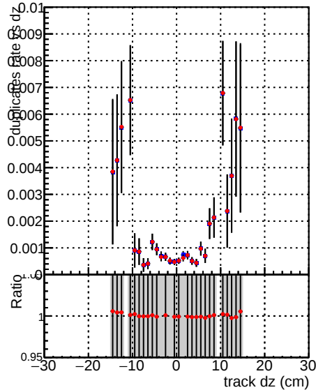
DQM CKF_XiMinusNOPU_base
