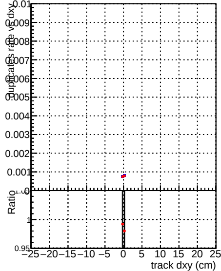
DQM CKF_XiMinusNOPU_base
