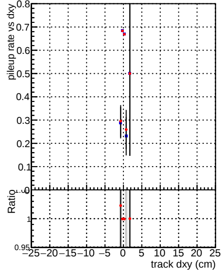
DQM CKF_XiMinusNOPU_retrainOldFiles125_v2_prelimWPM_epoch1
