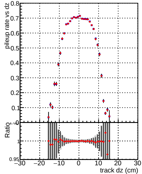
DQM CKF_XiMinusNOPU_retrainOldFiles125_v2_prelimWPM_epoch1
