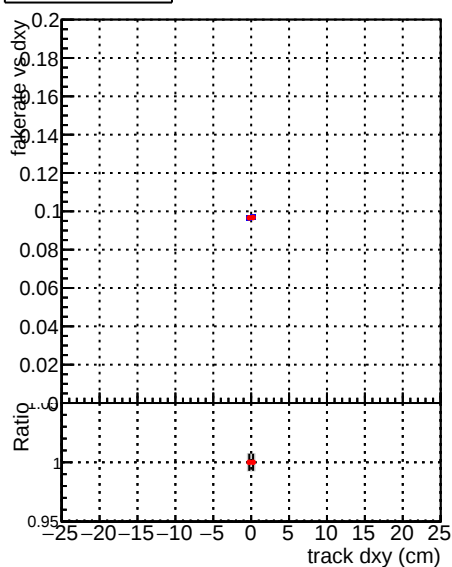
—•— DQM_CKF_XiMinusNOPU_base —•— DQM_CKF_XiMinusNOPU_retrainOldFiles125_v2_prelimWPM_epoch1
