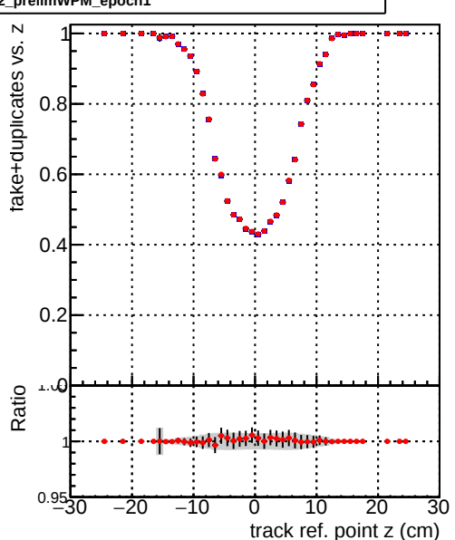
—•— DQM_CKF_XiMinusNOPU_base —•— DQM_CKF_XiMinusNOPU_retrainOldFiles125_v2_prelimWPM_epoch1
