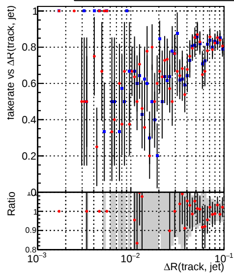
Legend: DQM_CKF_XiMinusNOPU_base DQM_CKF_XiMinusNOPU_retrainOldFiles125_v2_prelimWPM_epoch1
