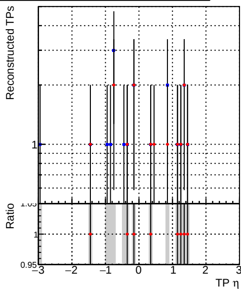
—•— DQM_CKF_XiMinusNOPU_base —•— DQM_CKF_XiMinusNOPU_retrainOldFiles125_v2_prelimWPM_epoch1
