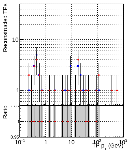
—•— DQM_CKF_XiMinusNOPU_base —•— DQM_CKF_XiMinusNOPU_retrainOldFiles125_v2_prelimWPM_epoch1
