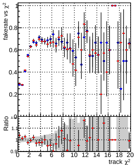
—●— DQM CKF XMinusNOPU_base —●— DQM CKF XMinusNOPU_retrainOldFiles125_v2_prelimWPM_epoch1
