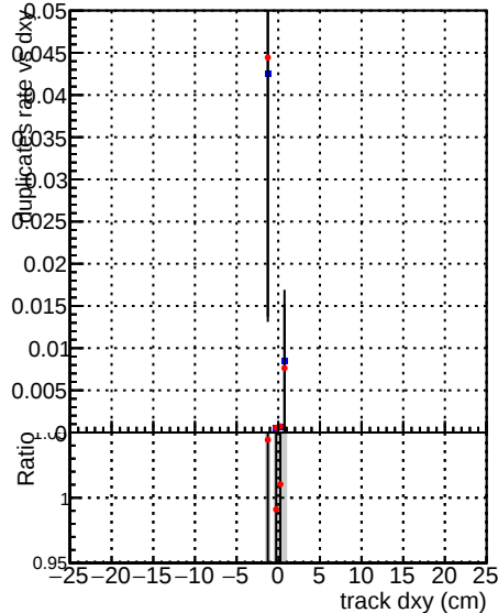
—●— DQM CKF_XiMinusNOPU_base —●— DQM CKF_XiMinusNOPU_retrainOldFiles125_v2_prelimWPM_epoch1
