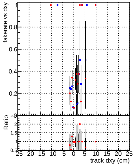
DQM CKF_XiMinusNOPU_retrainOldFiles125_v2_prelimWPM_epoch1
