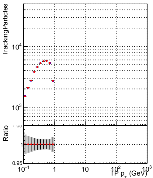
—●— DQM_CKF_XiMinusNOPU_base —●— DQM_CKF_XiMinusNOPU_retrainOldFiles125_v2_prelimWPM_epoch0
