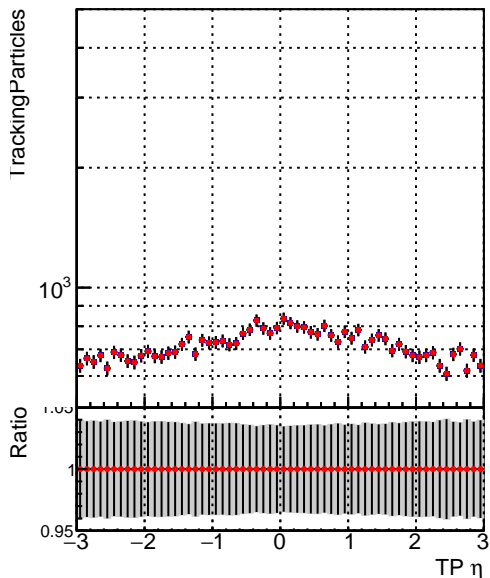
—●— DQM_CKF_XiMinusNOPU_base —●— DQM_CKF_XiMinusNOPU_retrainOldFiles125_v2_prelimWPM_epoch0
