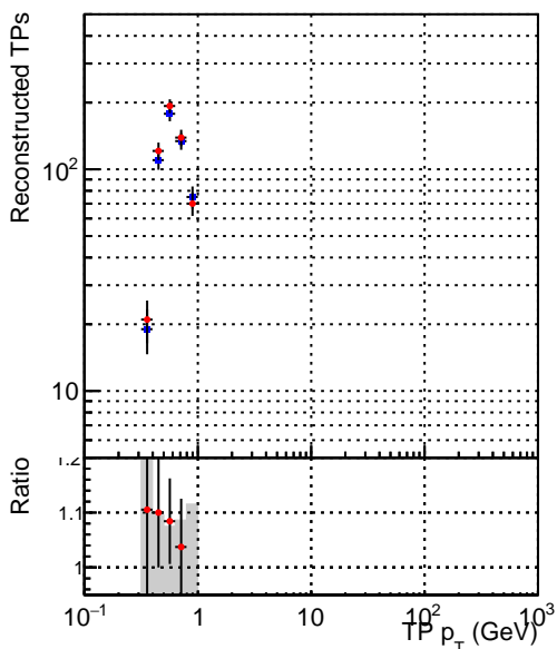
—●— DQM_CKF_XiMinusNOPU_base —●— DQM_CKF_XiMinusNOPU_retrainOldFiles125_v2_prelimWPM_epoch0
