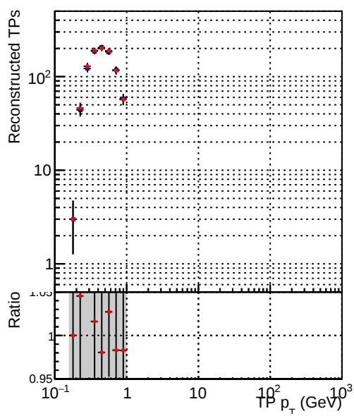
—●— DQM_CKF_XiMinusNOPU_base —◆— DQM_CKF_XiMinusNOPU_retrainOldFiles125_v2_prelimWPM_epoch0
