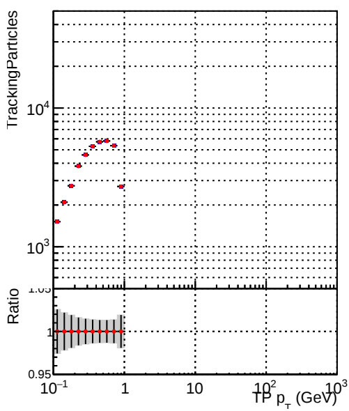
—●— DQM_CKF_XiMinusNOPU_base —◆— DQM_CKF_XiMinusNOPU_retrainOldFiles125_v2_prelimWPM_epoch0
