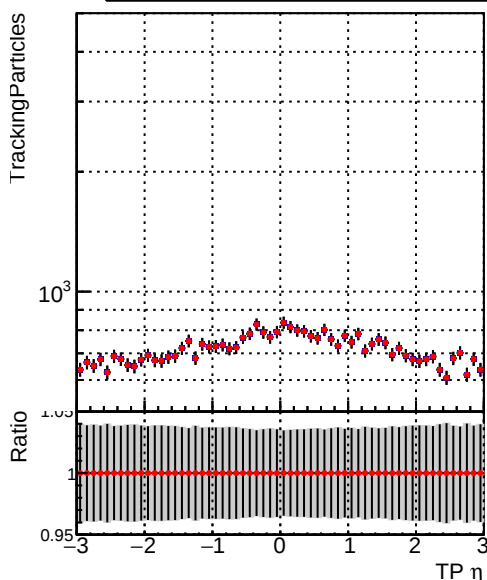
—●— DQM_CKF_XiMinusNOPU_base —◆— DQM_CKF_XiMinusNOPU_retrainOldFiles125_v2_prelimWPM_epoch0
