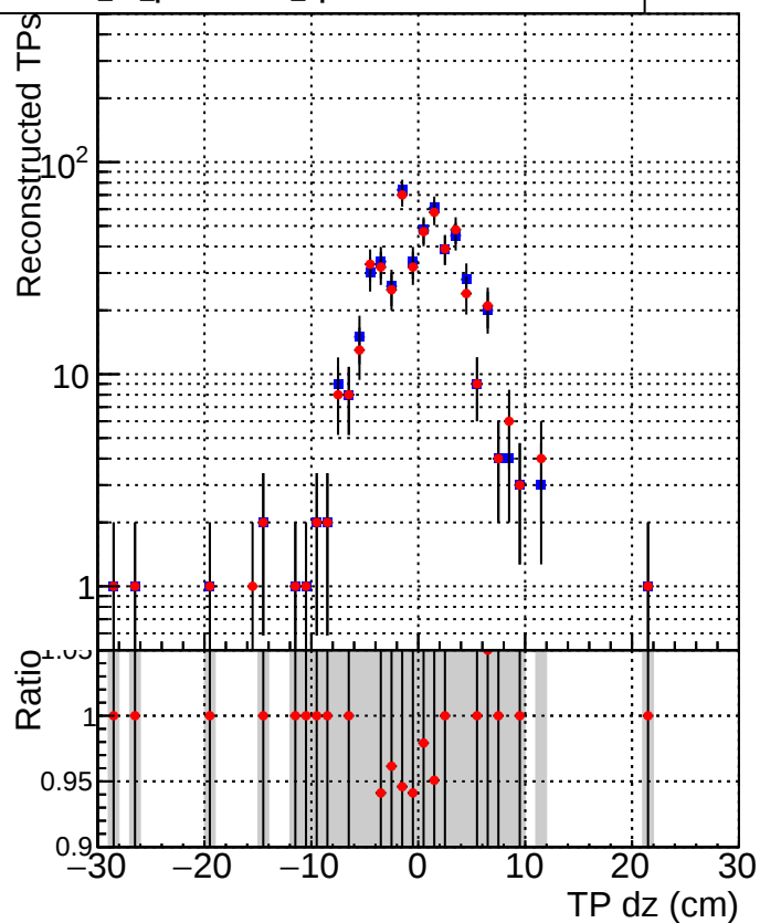
DQM_CKF_XiMinusNOPU_base DQM_CKF_XiMinusNOPU_retrainOldFiles125_v2_prelimWPM_epoch0
